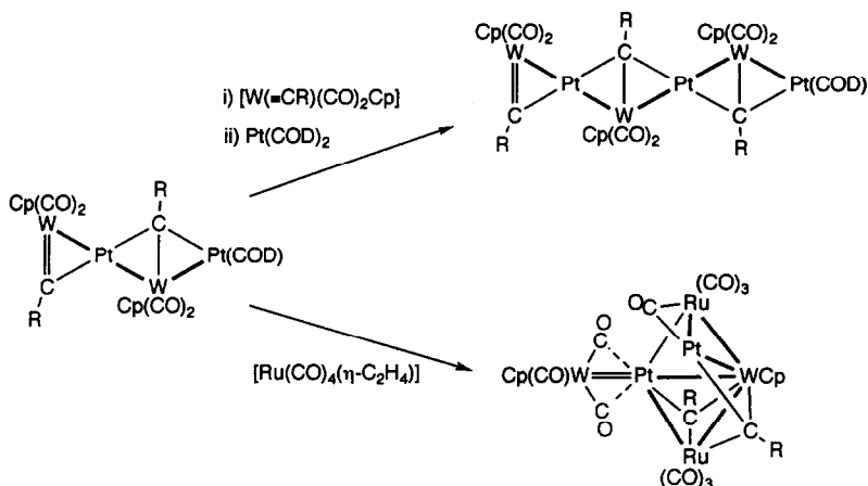
Scheme 16.
